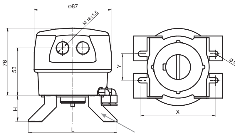
Dimensions GEMÜ 4221 [mm]
